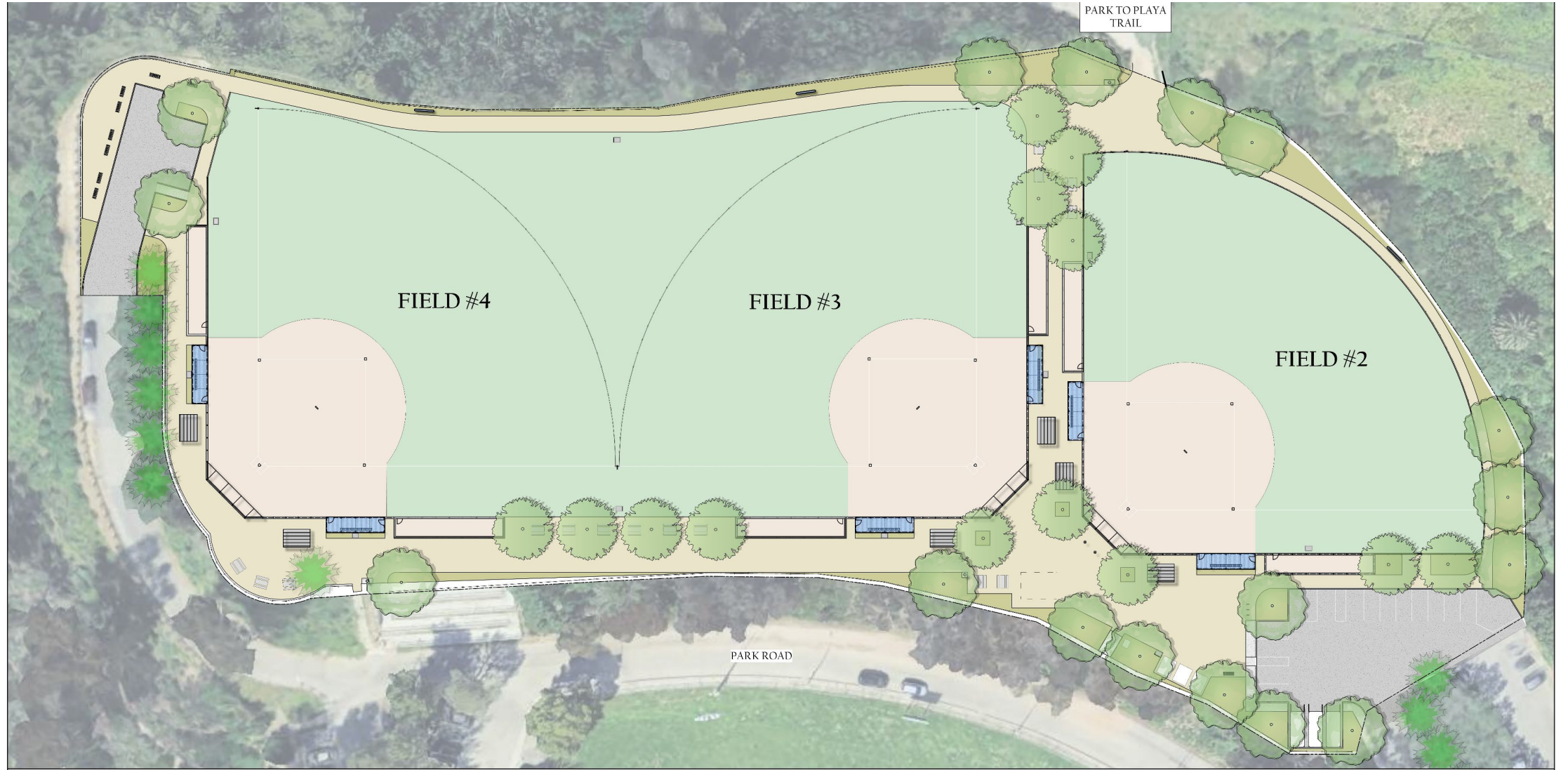
PARK PLAN Scale: 1:300
